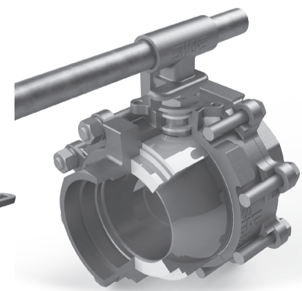
Válvula de Esfera com Cavidade Preenchida
