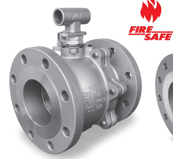
Válvula de Esfera Bipartida Flange Classe 150
