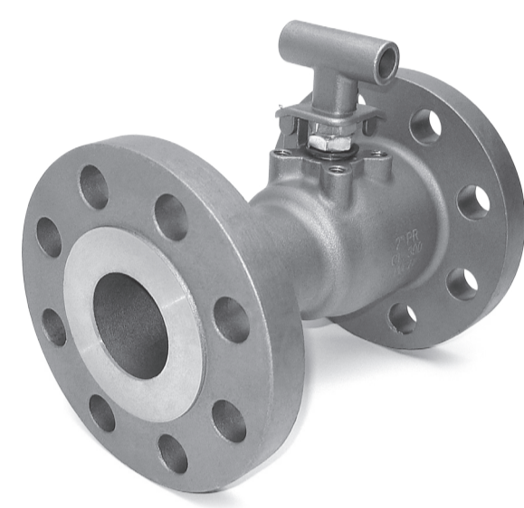
Válvula de Esfera Monobloco para Fundo de Caldeira Classe 150 / 300
