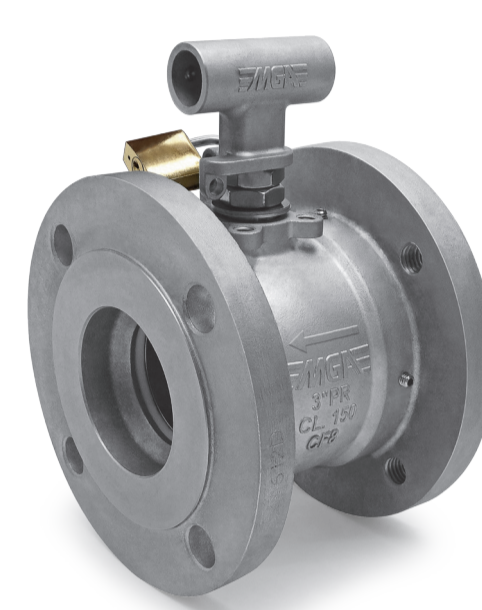
Válvula de esfera Wafer Flangeada Classe 150
