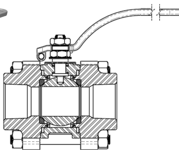
Figura 1 – Corte transversal da VET Classe 800
