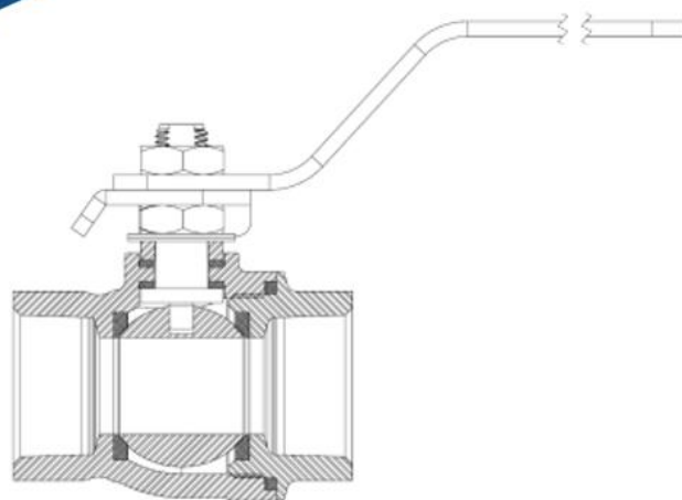
Figura 1 – Corte transversal
