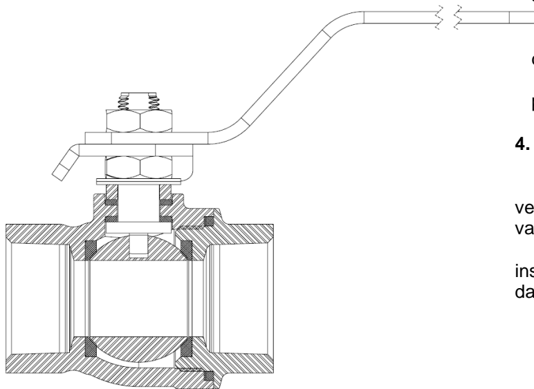
Figura 1 – Corte transversal da VEM Cl. 1000 WOG Montada.
